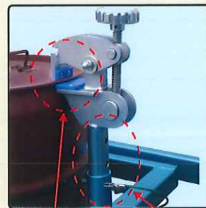
チャック 樹脂プレート取り付け
