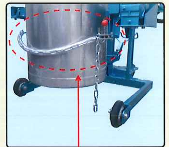
5段階 伸縮チャック
